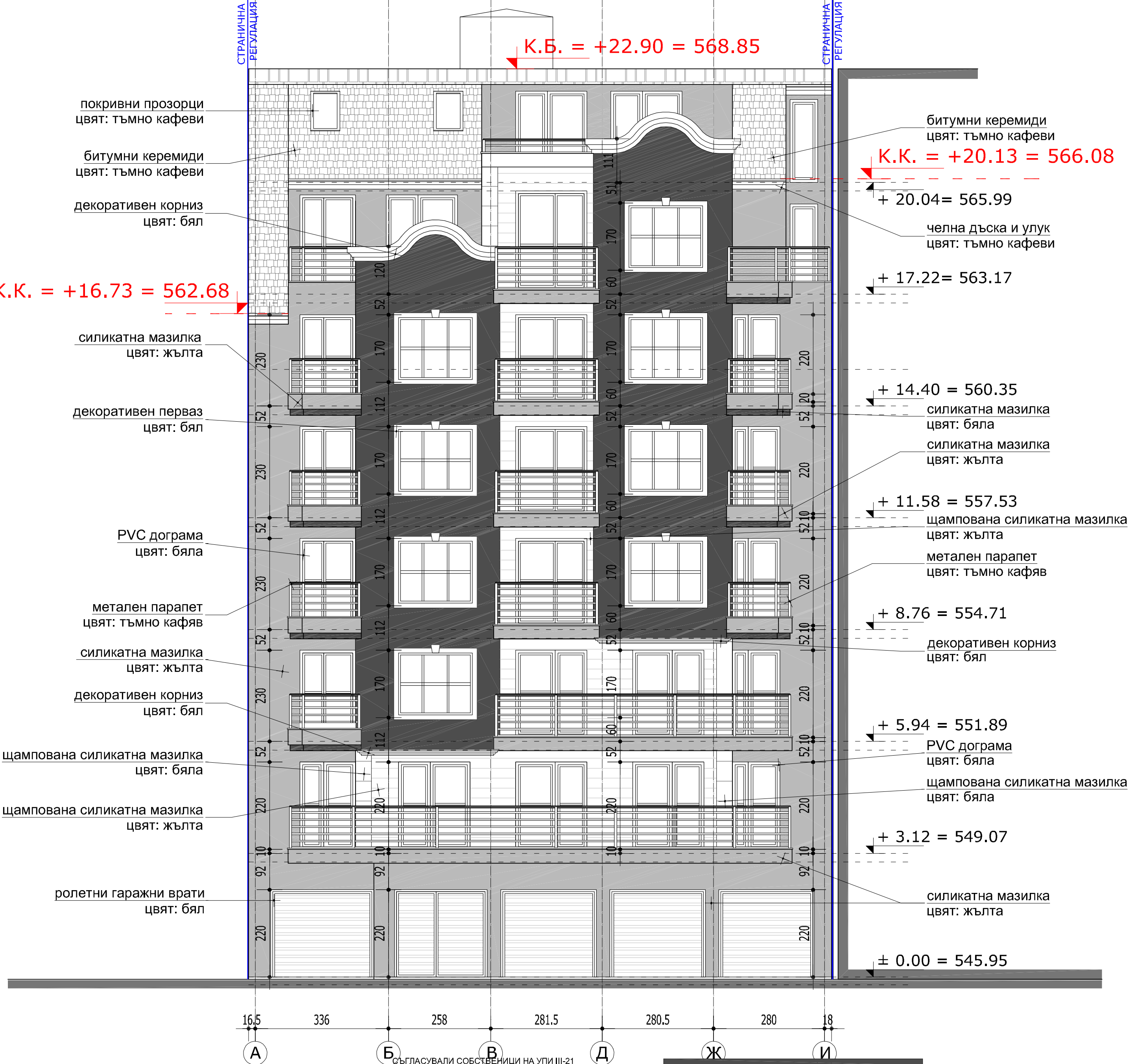
ФАСАДА ЗАПАД М1:75
