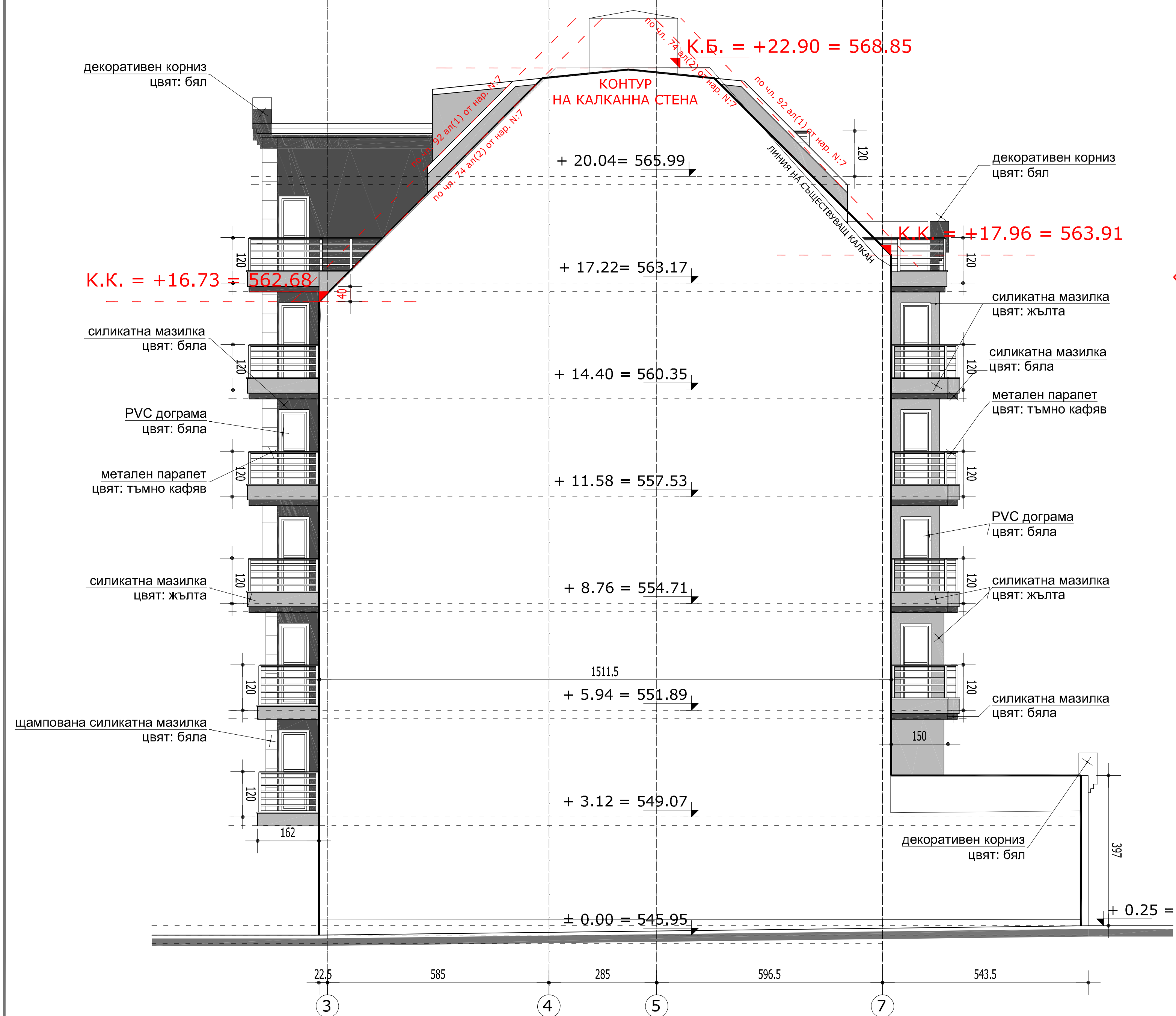
КАЛКАН ФАСАДА ЮГ М1:75
