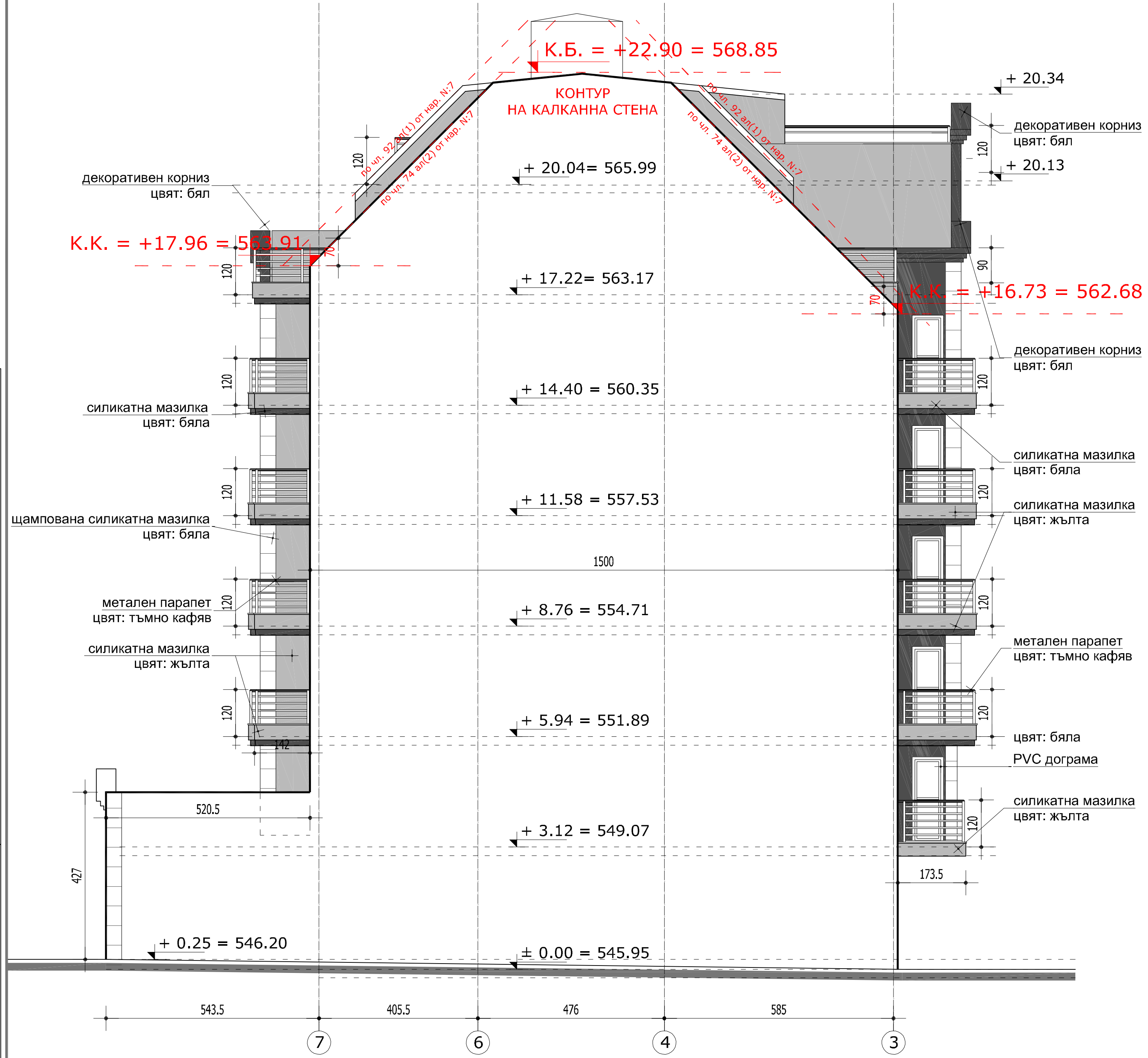
КАЛКАН ФАСАДА СЕВЕР М1:75
