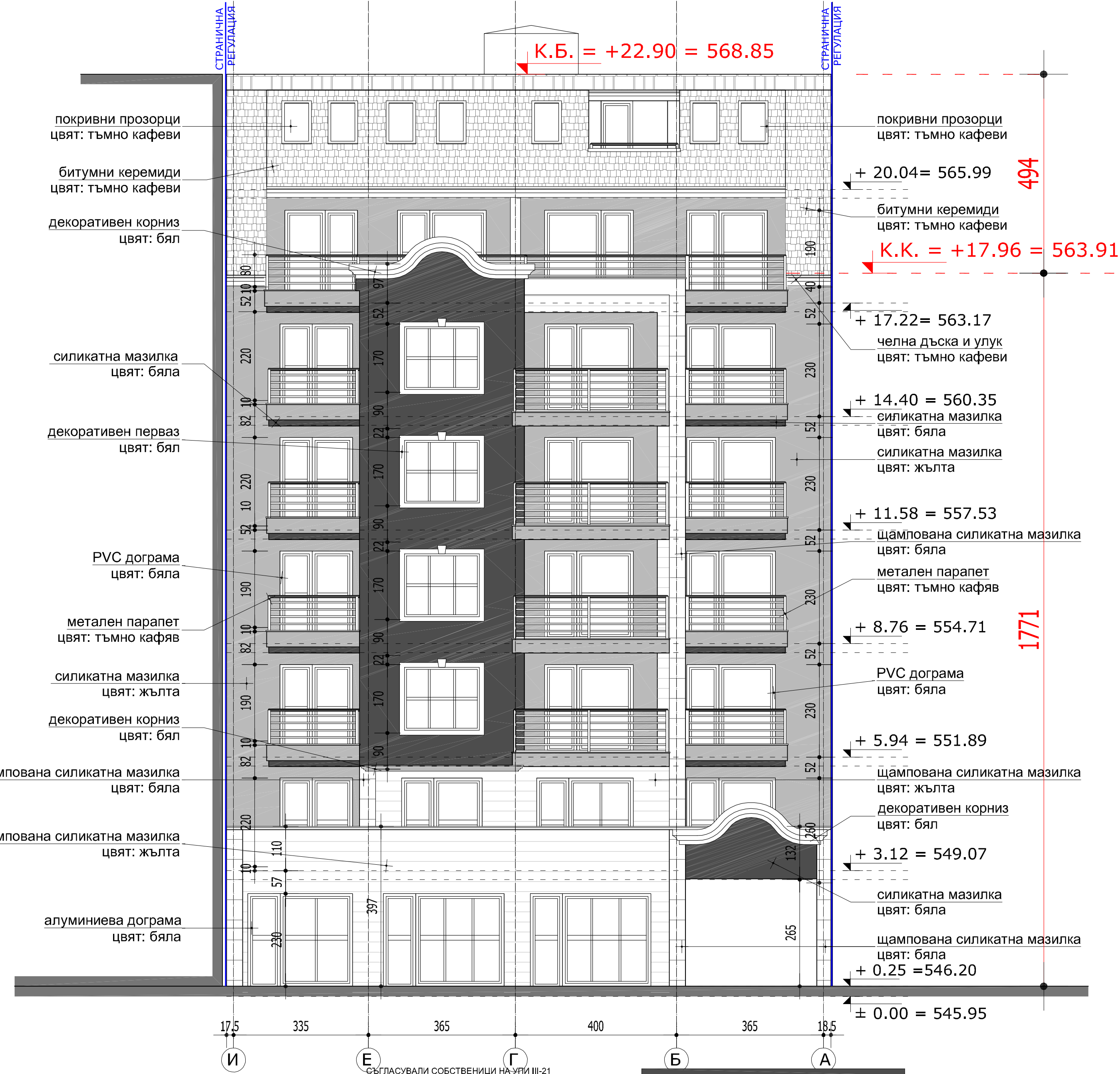
ФАСАДА ИЗТОК М1:75
